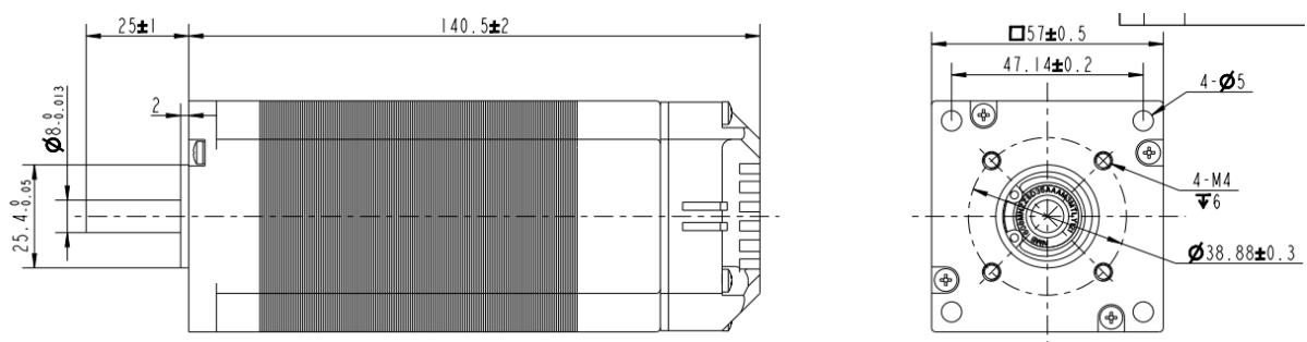
图 1 机械尺寸图
